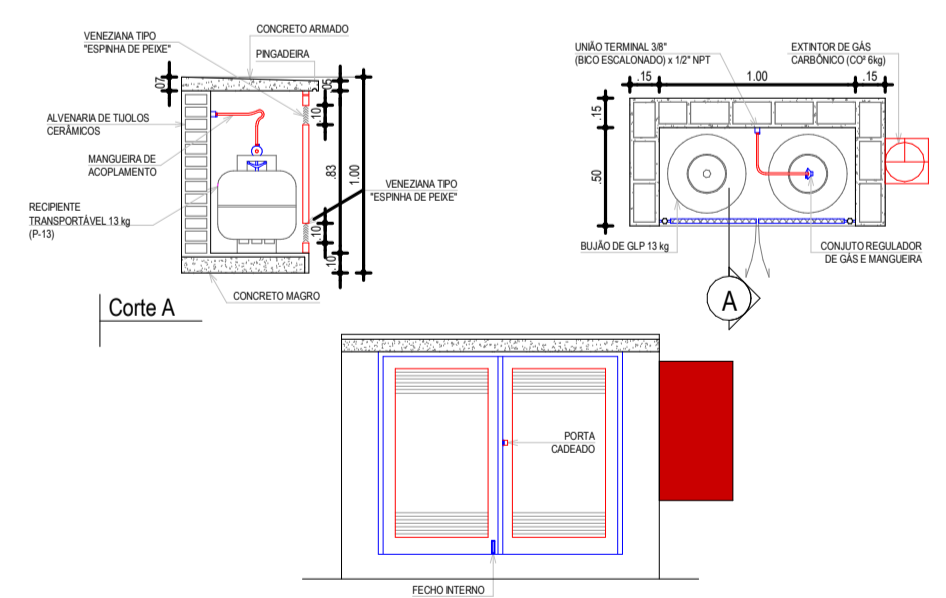
DETALHE CENTRAL DE GÁS GLP S/ ESCALA
