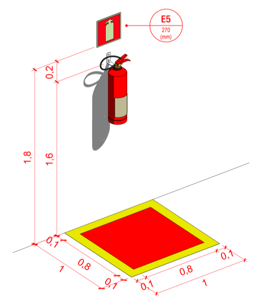
DETALHE EXTINTOR PAREDE - 3D S/ ESCALA
