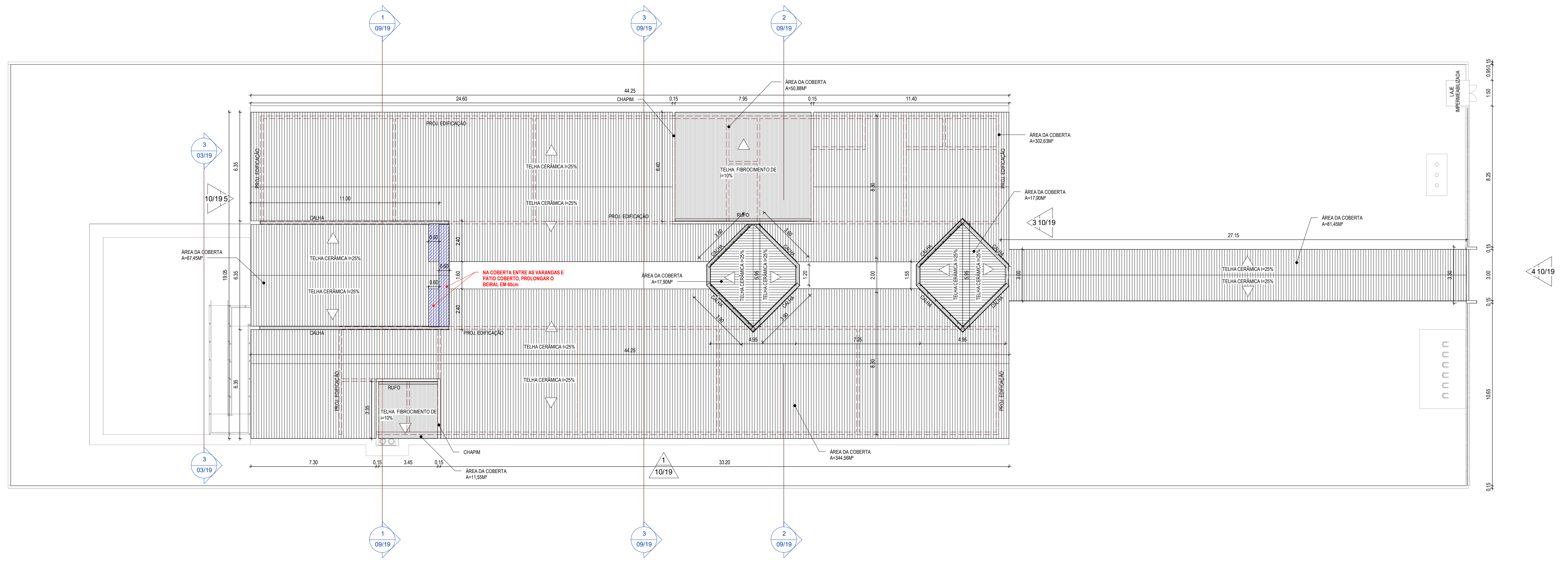
1 PLANTA DE COBERTA 1 : 125
