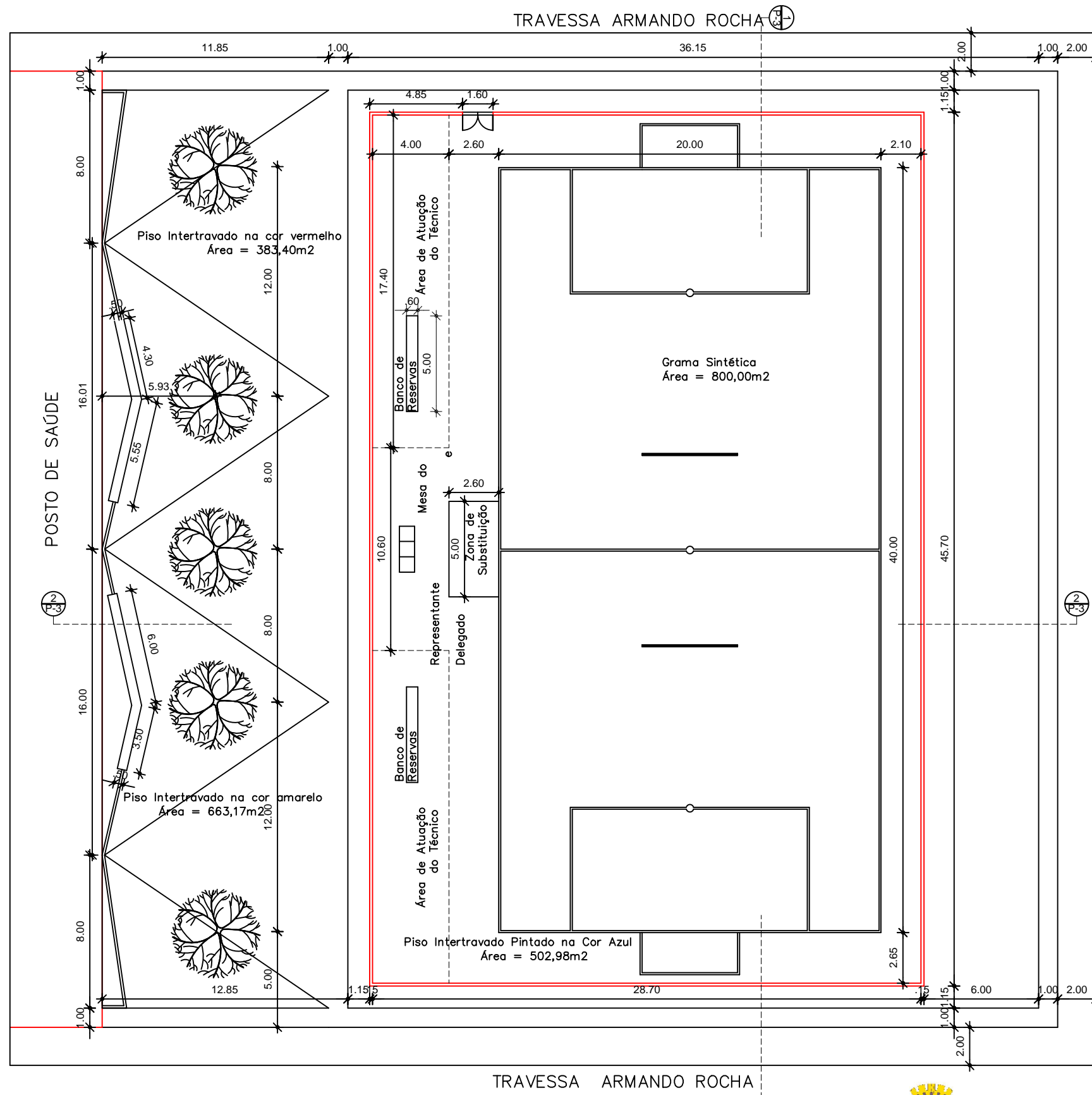
1 PLANTA BAIXA ARENINHA PEDREGAL ESC. 1/250
