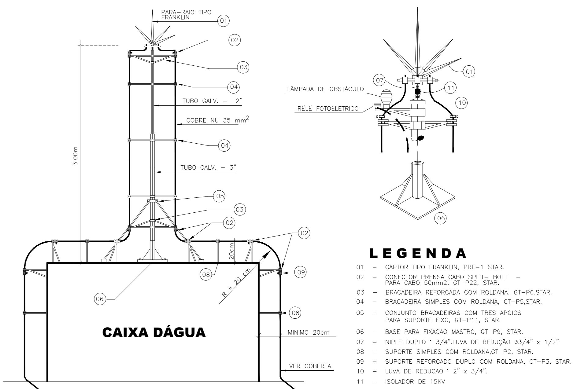
DETALHE DO PARA-RAIOS TIPO FRANKLIN SEM ESCALA
