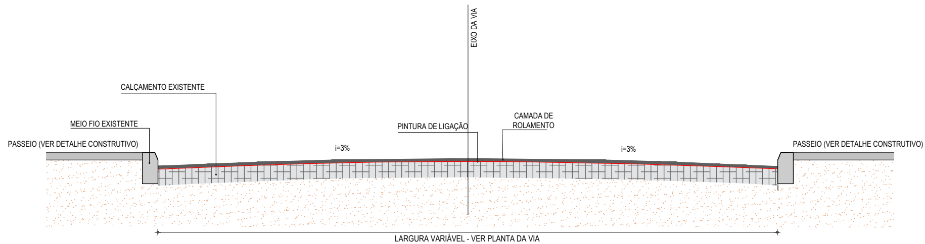
SEÇÃO TIPO ESCALA: SEM ESCALA
