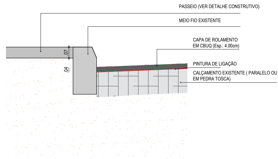
DETALHE DOS MATERIAIS SEM ESCALA
