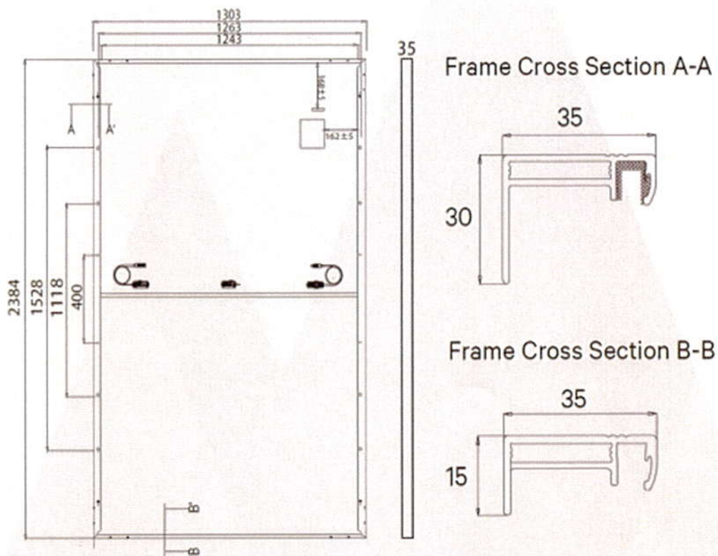
Figura 05: Modelo do módulo fotovoltaico.
