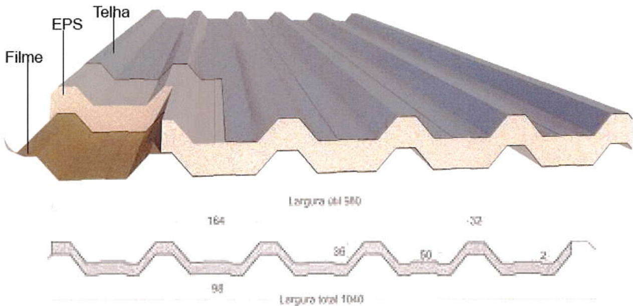
Figura 04: Imagem esquemática da telha termoacústica trapezoidal.
