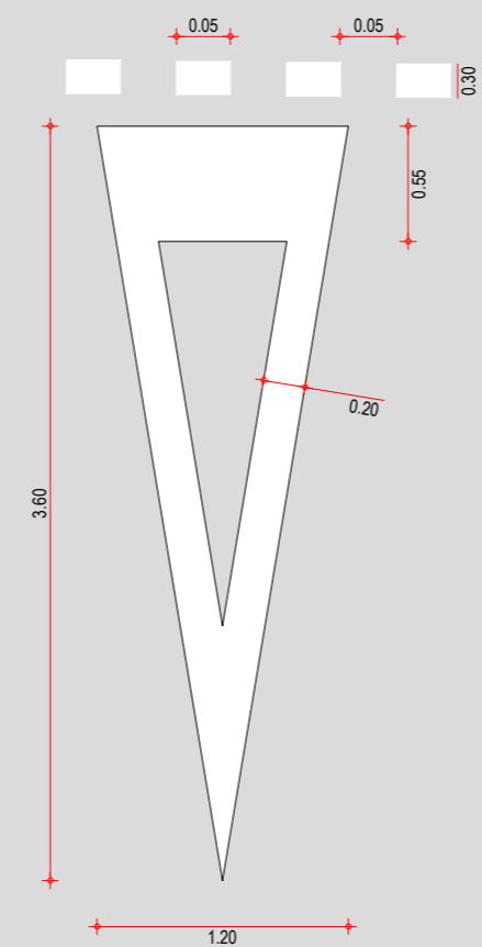
DETALHE 3 SIMBOLO: DE A PREFERÊNCIA
