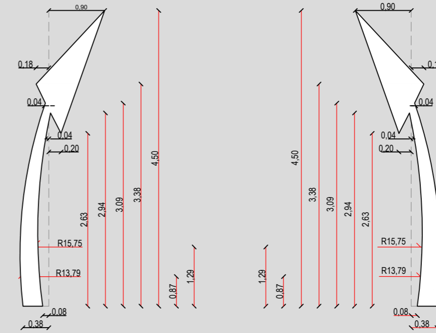
DETALHE 4 SETAS INDICATIVAS DE MOVIMENTOS EM CURVA (IMC)
