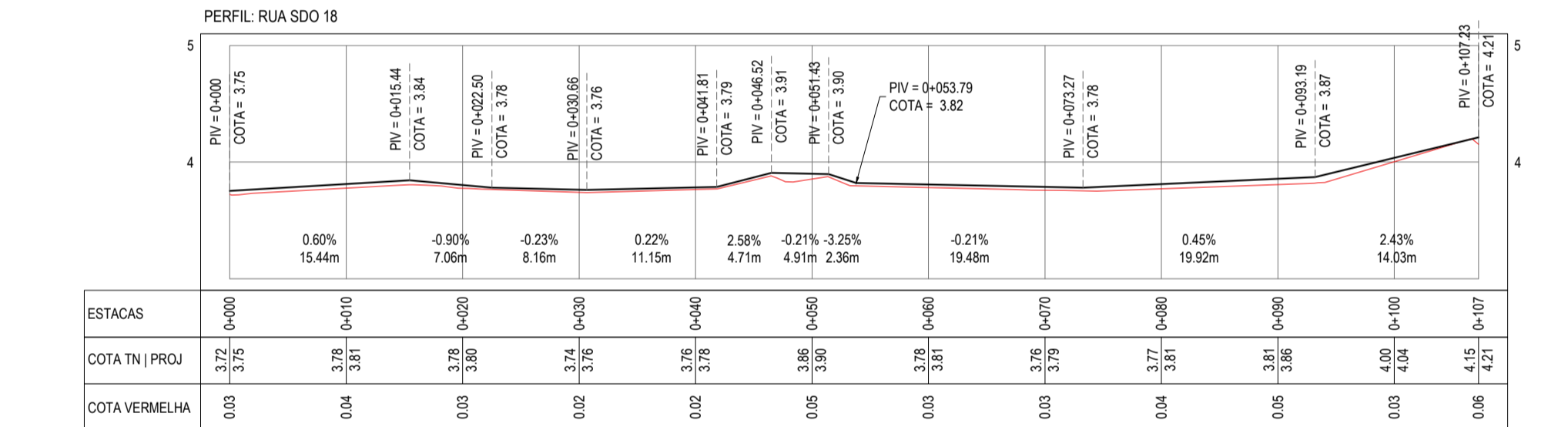
PERFIL LONGITUDINAL RUA SDO 18 ESCALA: H 1/750 | V 1/750
