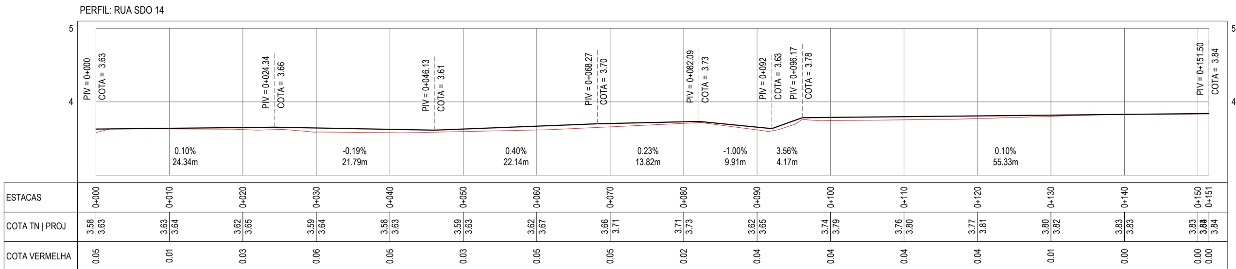
PERFIL LONGITUDINAL RUA SDO 14 ESCALA: H 1/750 | V 1/750
