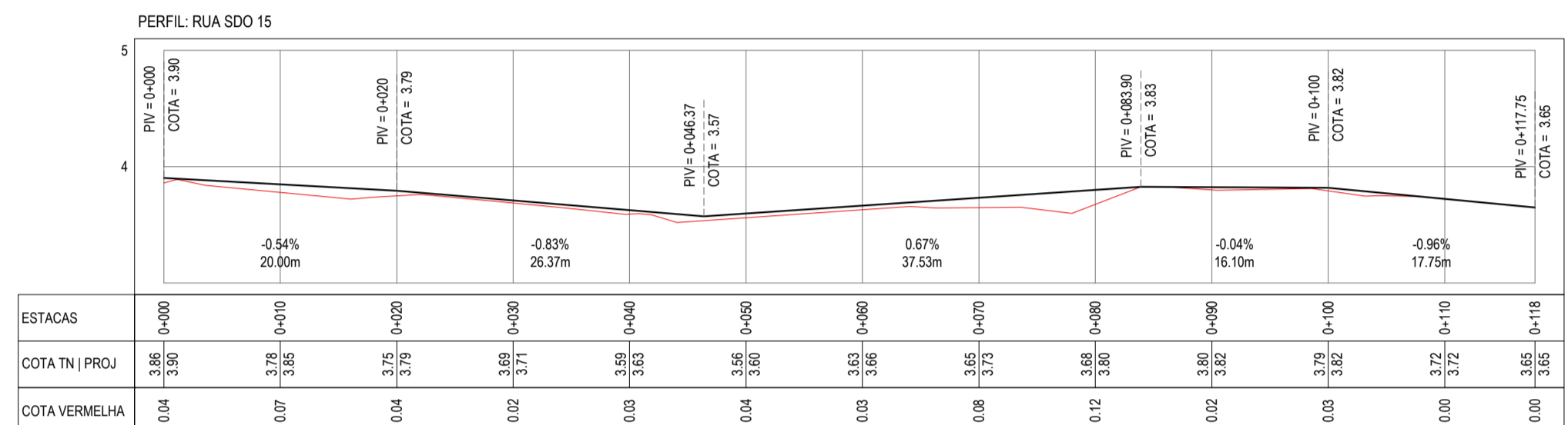
PERFIL LONGITUDINAL RUA SDO 15 ESCALA: H 1/750 | V 1/750
