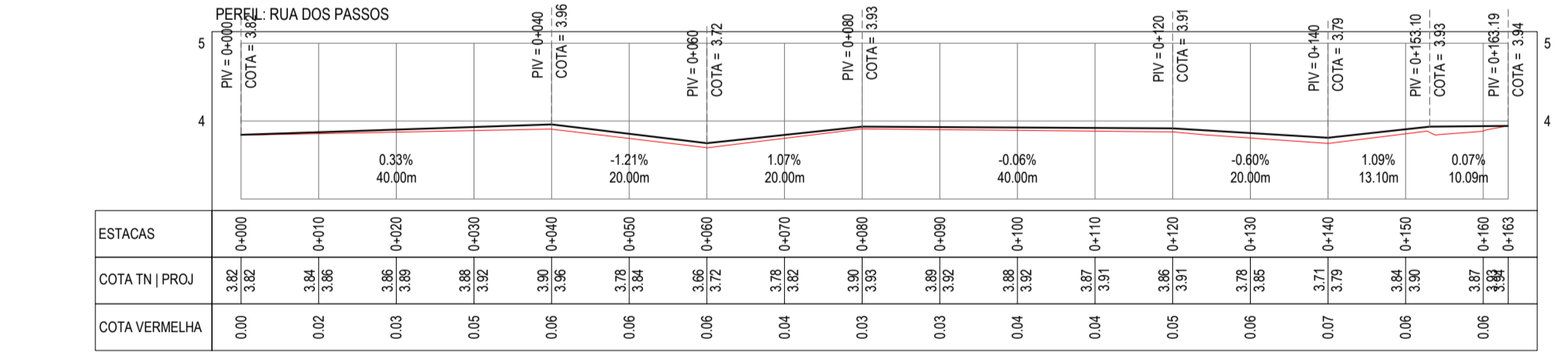
PERFIL LONGITUDINAL RUA DOS PASSOS ESCALA: H 1/750 | V 1/750
