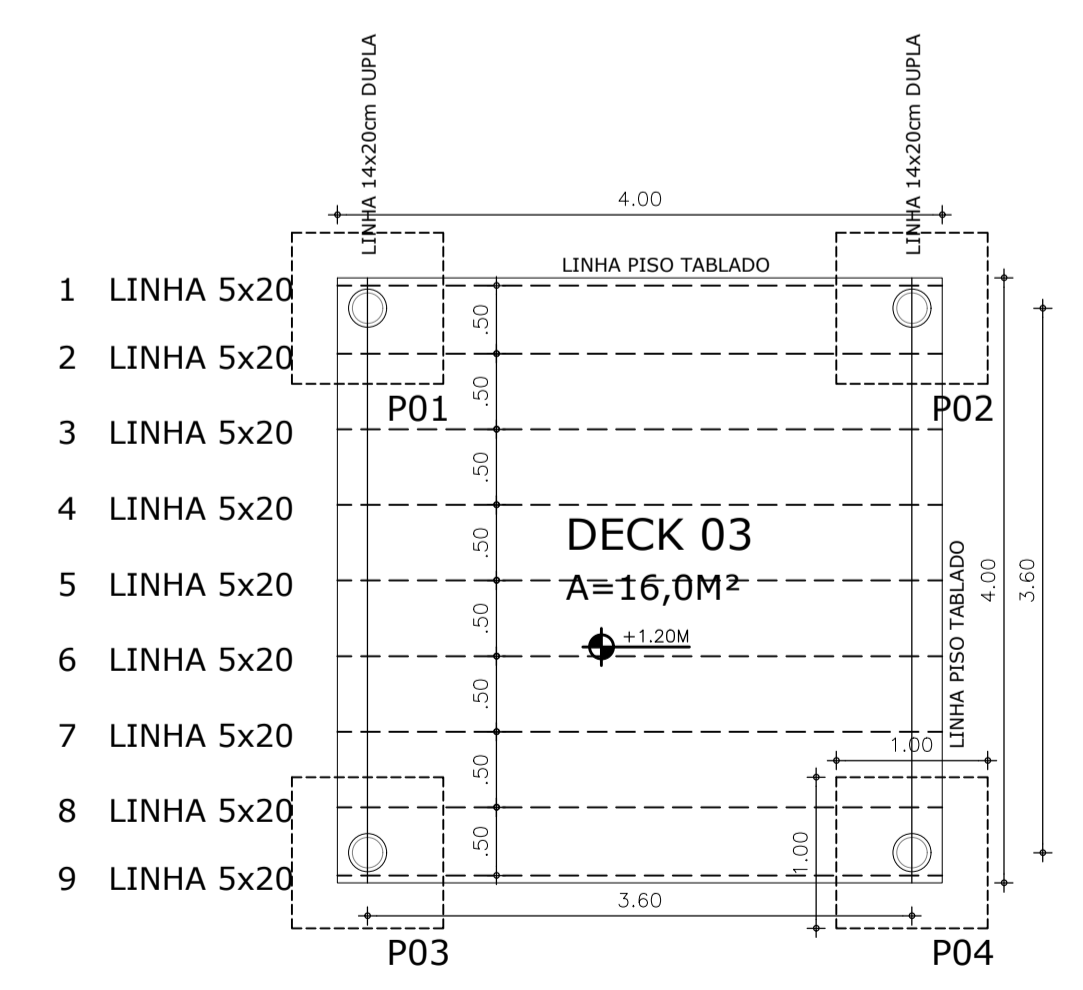
PLANTA BAIXA COTAS SAPATAS/LINHAS DECK 03 1-50
