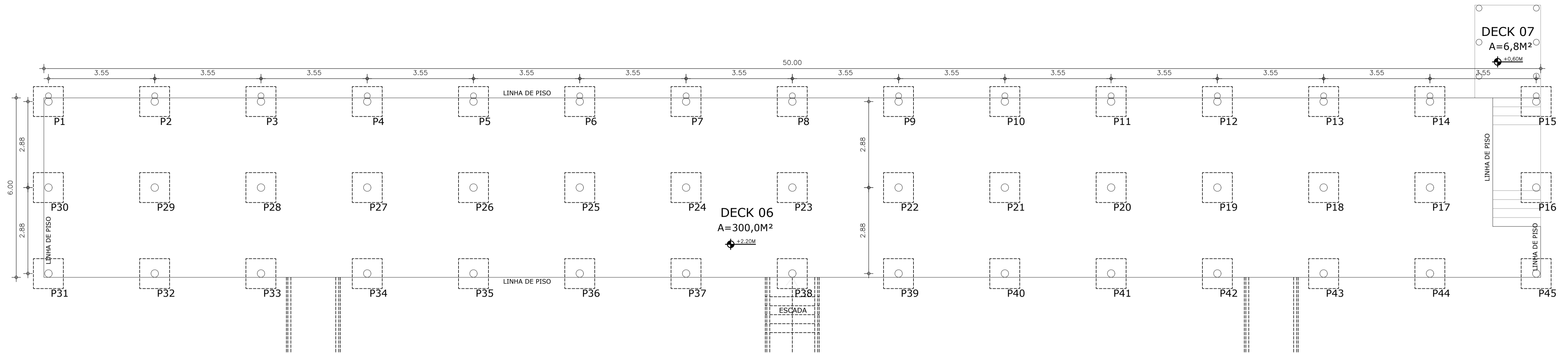
PLANTA BAIXA LOCAÇÃO SAPATAS DECK 06 1-75
