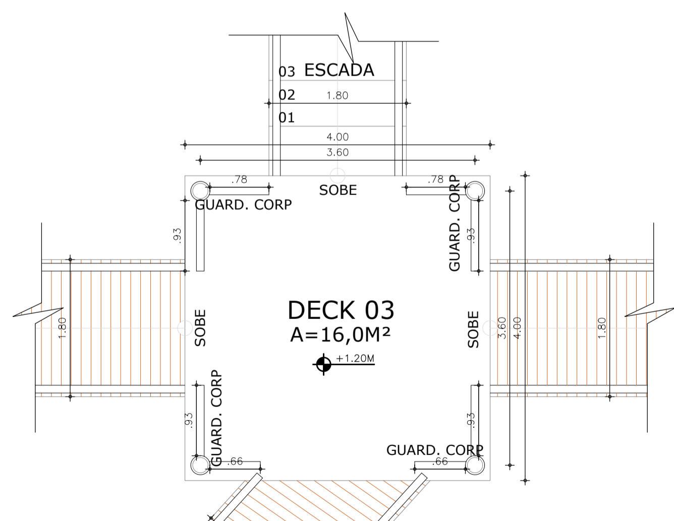
PLANTA BAIXA COTAS DECK 03 1-50
