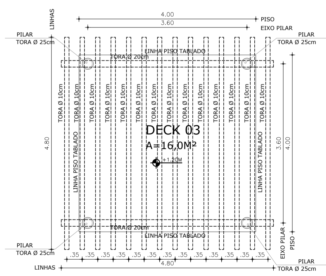
PLANTA BAIXA PERGOLADO COTAS DECK 03 1-50
